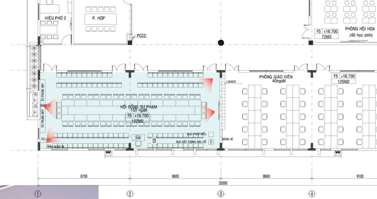
MẶT BẰNG BỐ TRÍ VẬT DỤNG TẦNG 5 TL: 1/100
